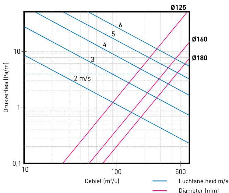
Drukverlies per meter (in verhouding tot lichtsnelheid) - rechte uitvoering
