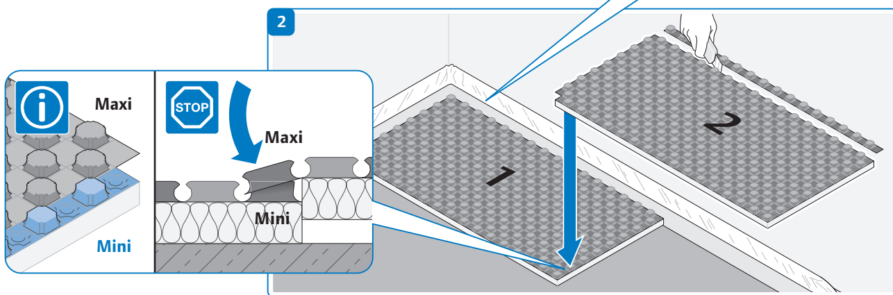
Noppenplaten monteren
